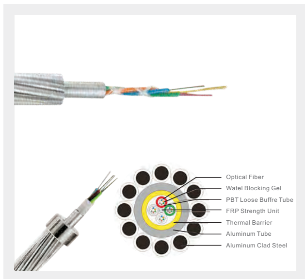
▲ OPGW cable
